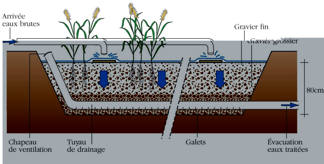
Figure 1 : Coupe transversale schématique d'un filtre à écoulement vertical 1
