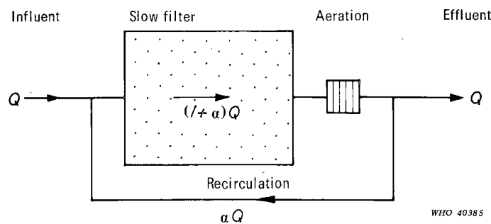
FIG. 23. RECIRCULATION OF EFFLUENT
