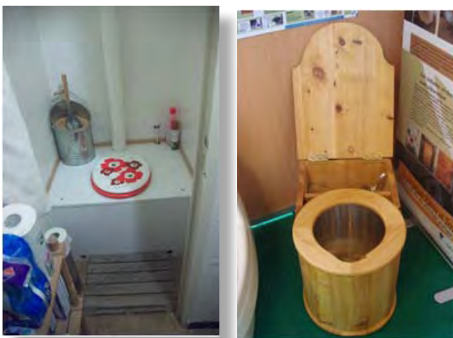
(à gauche) Toilettes sèches unitaires pour une famille avec réceptacle de 80 l
