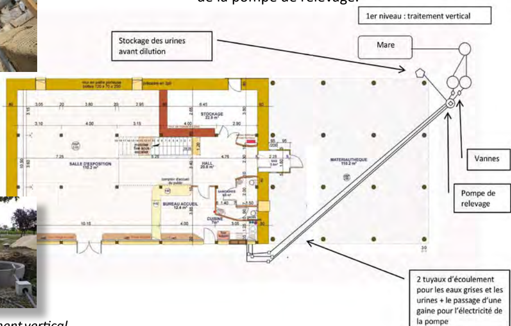
Premier niveau de traitement vertical aérobie posé sur le sol existant
