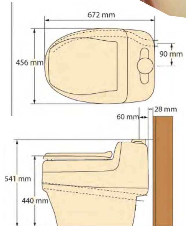
Côte d'englobement d'un separett villa 9000
