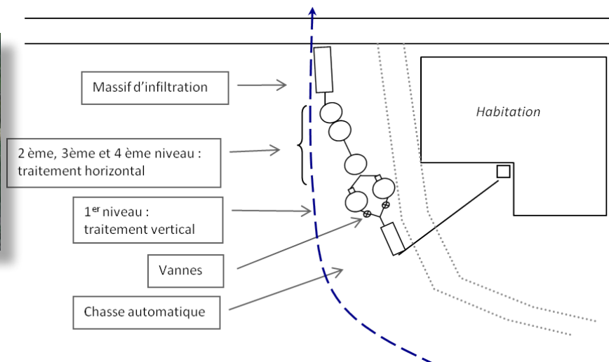
Premier niveau de traitement vertical aérobie fonctionnant en alternance et par bâchée
