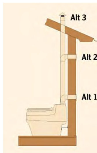
Schéma d'installation du Separett villa 9000
