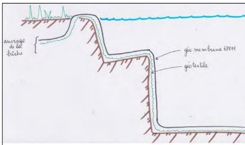
Schéma d'ancrage de la bâche
