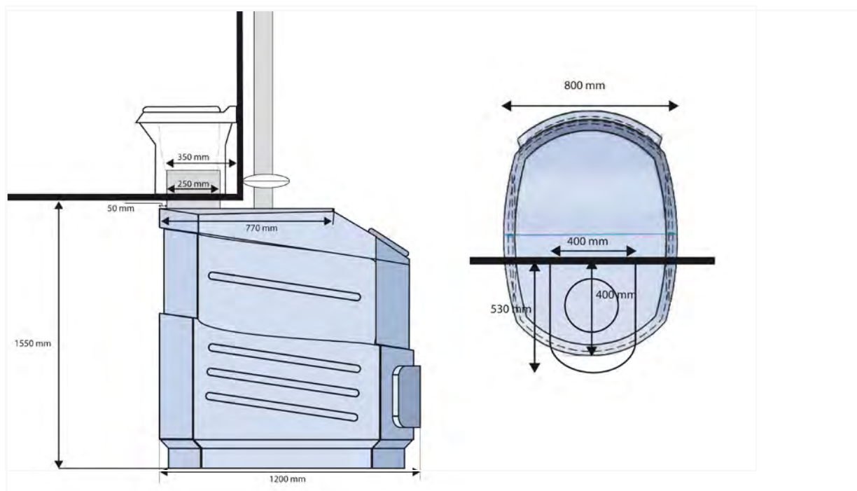
Positionnement du composteur Clivus
