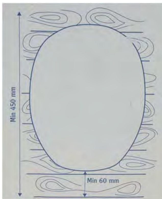
Schéma d'implantation du séparateur
