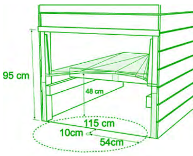
Schéma d'implantation de toilettes sèches unitaire VU de chez Ekolet
