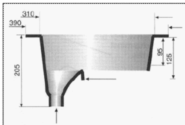
Mesures/coupe du séparateur d'urine
