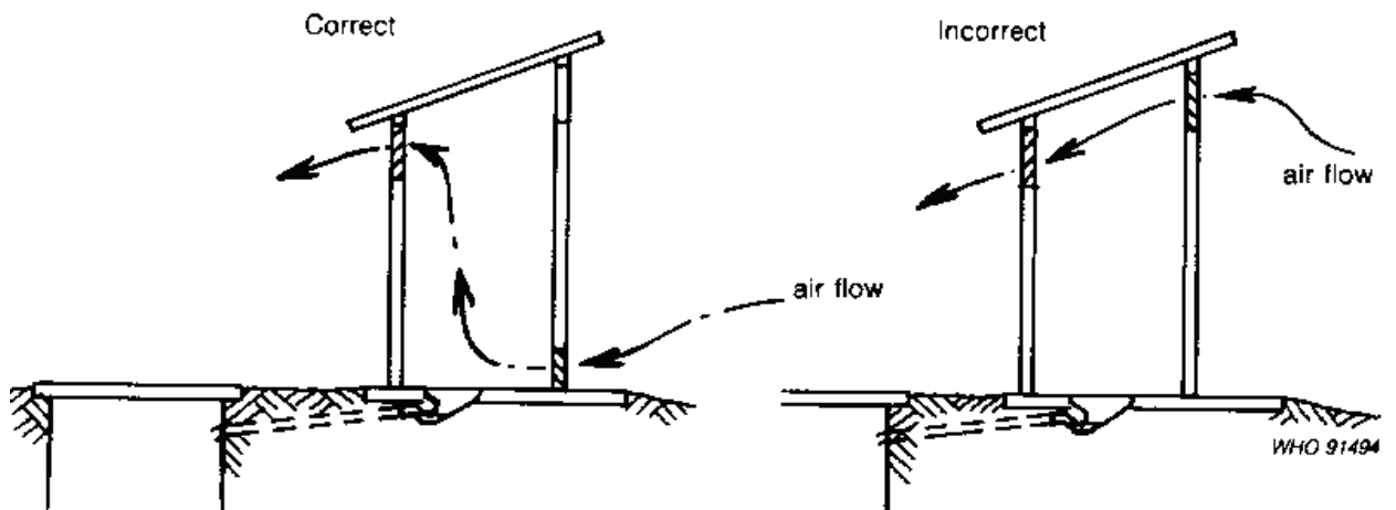
Fig. 7.34. Ventilation In a pour-flush latrine
