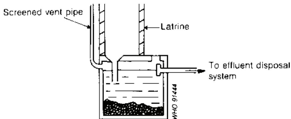
Fig. 6.25. Aqua-privy
