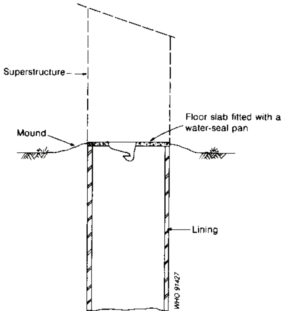
Fig. 6.8. Pour-flush latrine
