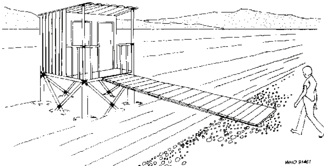
Fig. 6.42. Overhung latrine
