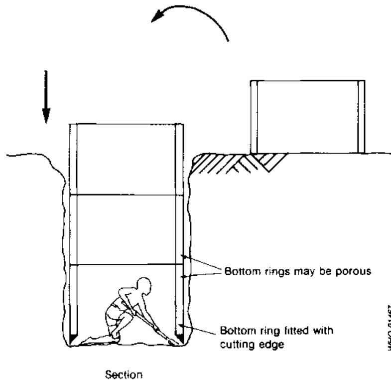
Fig. 7.7. "Caissoning" a pit
