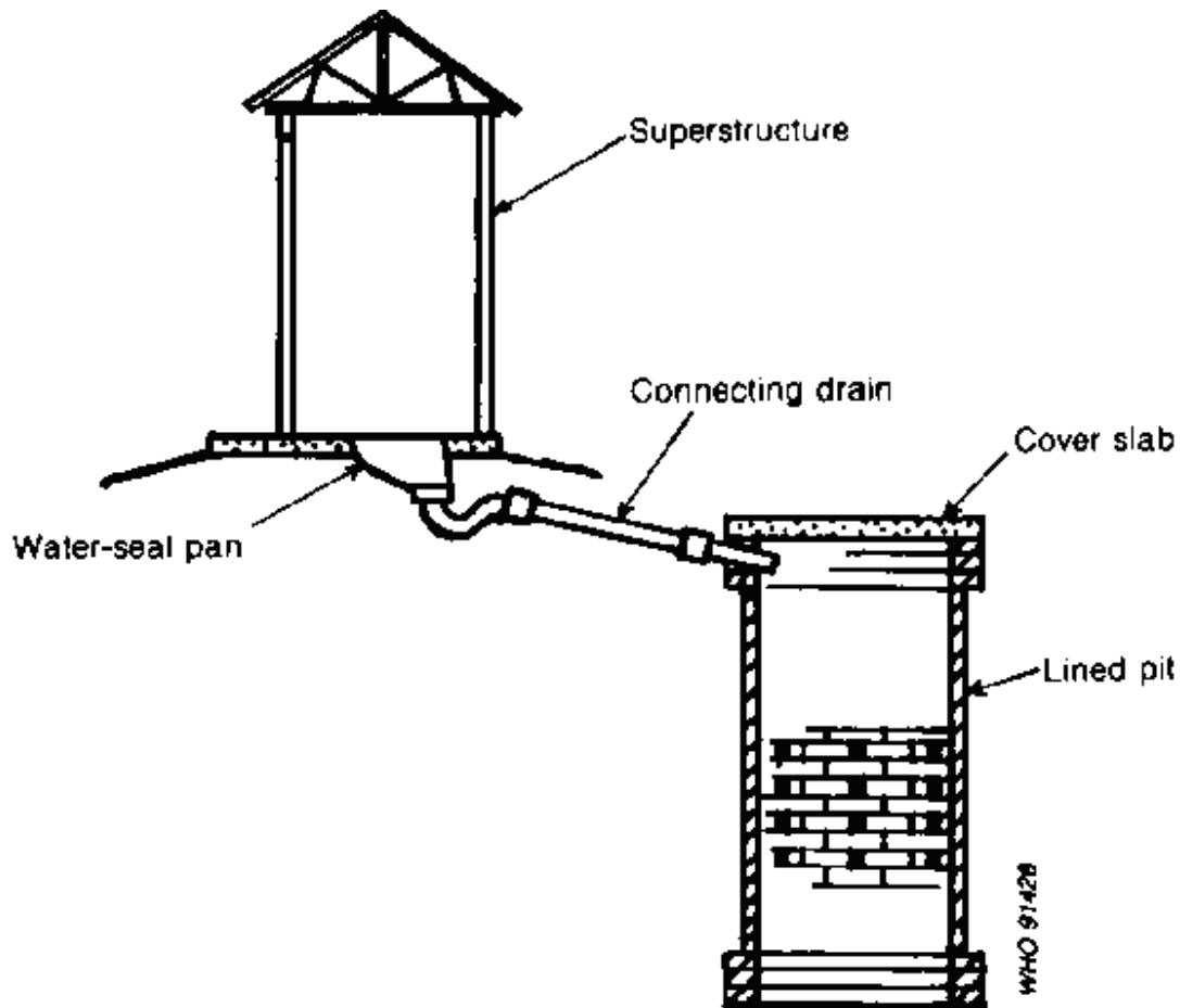
Fig. 6.9. Offset pour-flush latrine
