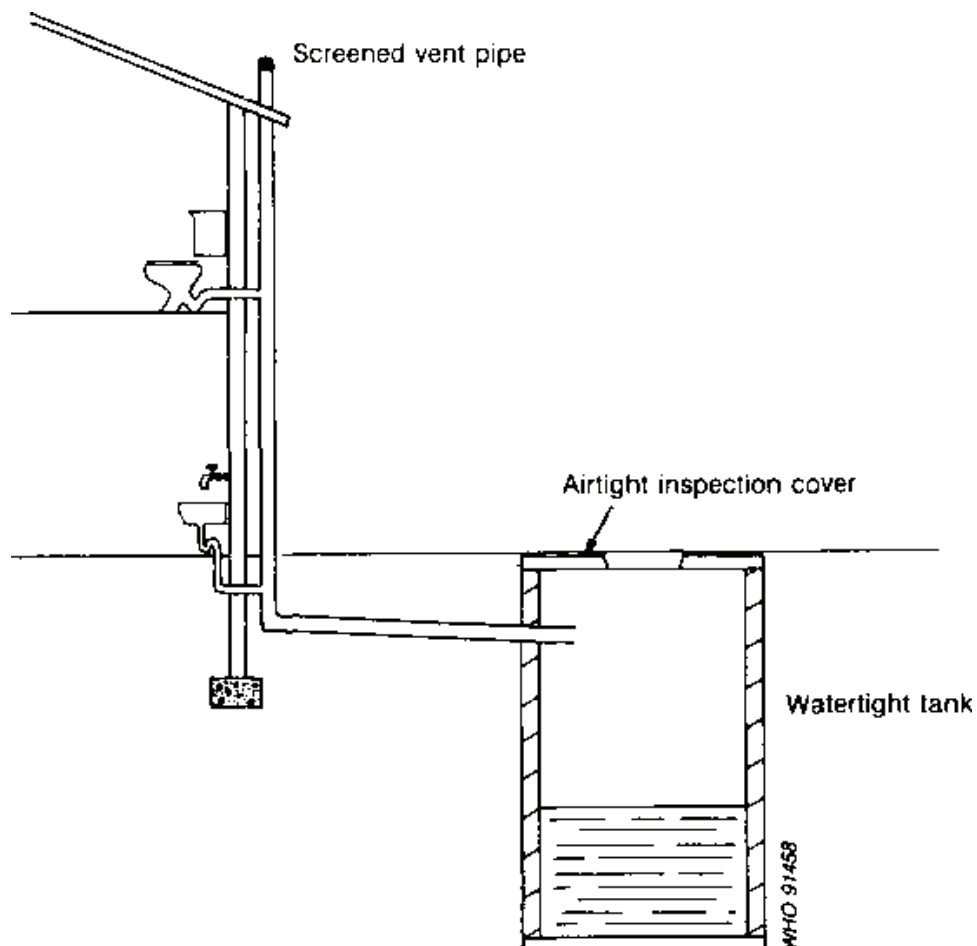
Fig. 6.39. Cesspit
